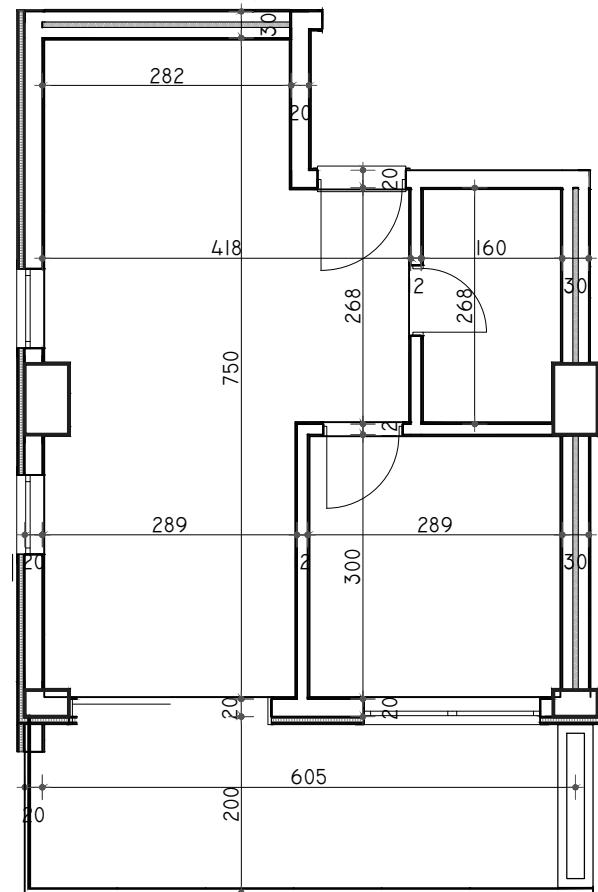
PLANIMETRIA E APARTAMENTIT - PERMASIM
